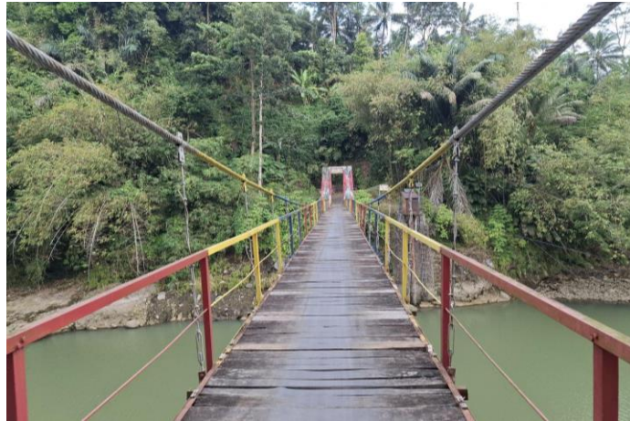
Gambar 12. Jembatan Gantung
